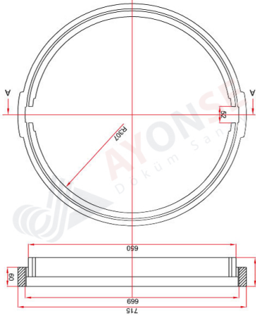
A-A Kesiti
